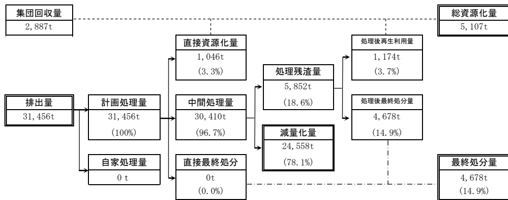
図2 目標達成時の一般廃棄物の処理状況フロー (平成 33 年度)
